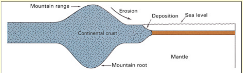
Apẹẹrẹ 9: apejuwe miran ti o fi han bi awọn oke se da gege bi eekan nibi aworan, nitoripe wọn ni awọn gbongbo jijin. (Earth Science. Tarbuck and Lutgens, P.158)
