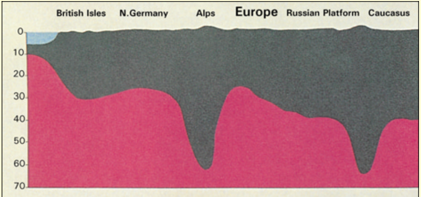
Apẹẹrẹ 8: ipin ilana: awọn oke da gege bi awọn eekan, wọn ni awọn gbongbo jijin labele. (Anatomy of the earth, Cailleux, p.220).S
