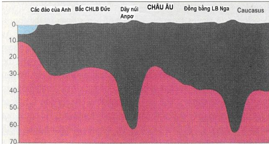
Hình 8. Mặt cắt ngang. Những ngọn núi giống như những cái cọc có chân cắm sâu vào lòng đất ( Anatomy of the Earth , Cailleux, trang 220)
