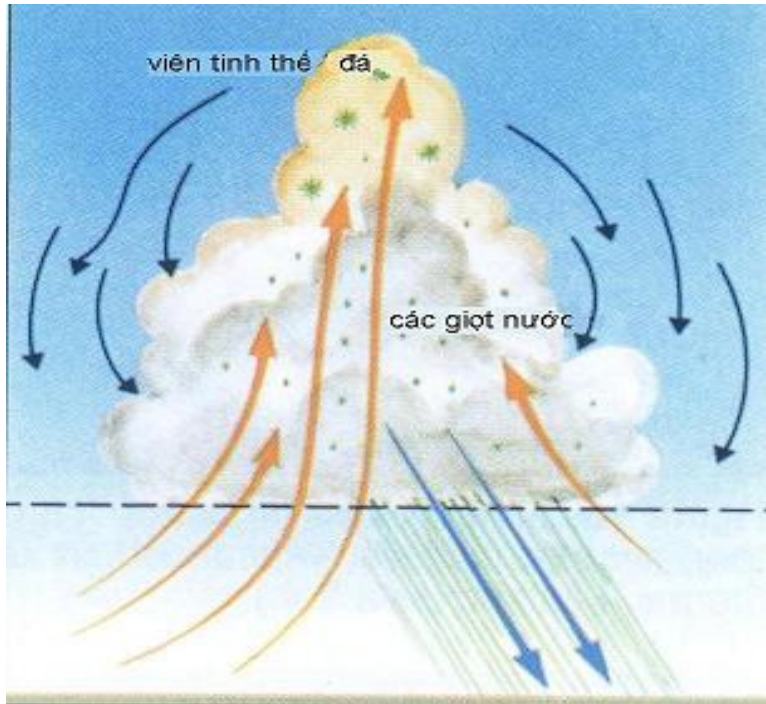
Hình 20. Một đám mây tích mưa. Sau khi mây được chòng cao lên, mưa rơi xuống từ đây ( Thời tiết và khí hậu , Bodin, trang 123).
