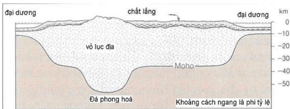
Hình 7. Các ngọn núi có rễ ăn sâu vào trong lòng đất ( Trái đất , Press and Siever, p.413)
