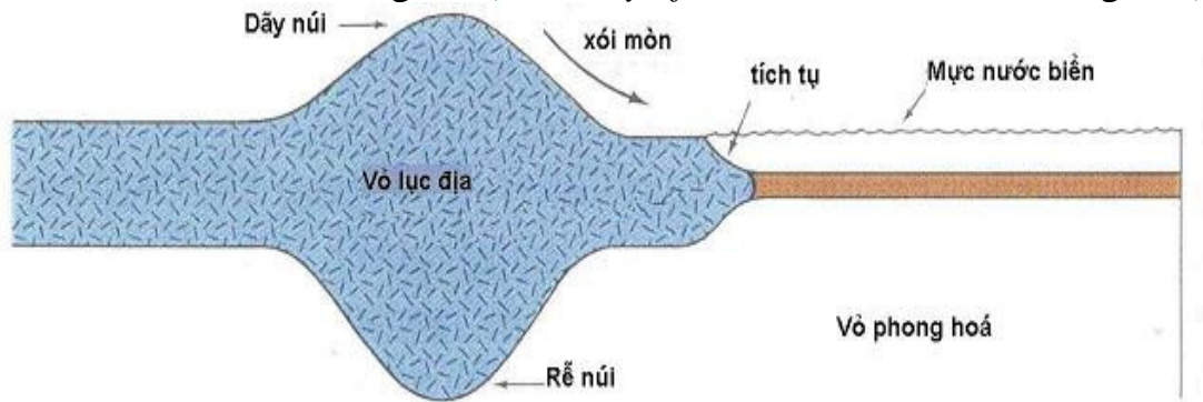
Hình 9. Minh họa khác cho thấy ngọn núi trông giống cái cọc như thế nào về hình dáng, vì chúng có rễ sâu ( Khoa học trái đất , Tarbuck và Lutgens, trang 158).
