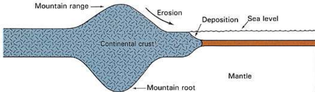
चित्र ९ : गहिरा जराहरूको कारणले चुकुल (Peg) जस्तो आकार लिएको पर्वत हरू देखाउने अर्को चित्र ( "Earth Science" Tarbuck & Lutgens , पृ.सं. १५८)
