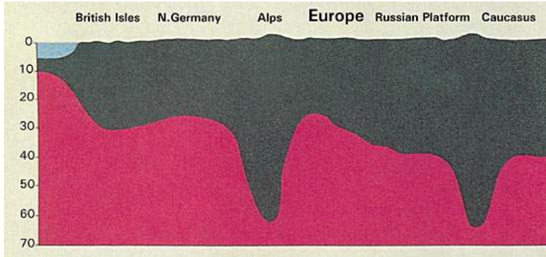
चित्र ८ : पर्वत का जमीनमा गाडिएका चुकुल (Peg) जस्ता जराहरू ( Anatomy of the Earth Cailleux , पृ.सं. २२०)
