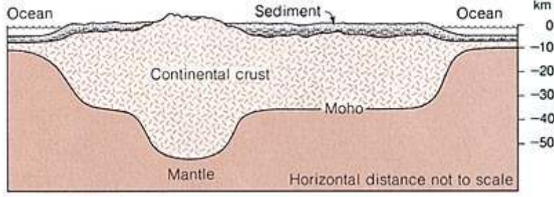
चित्र ७ : पर्वत का गहिरा जराहरू ( Earth, Press & Siever , पृ.सं. ४१३)
