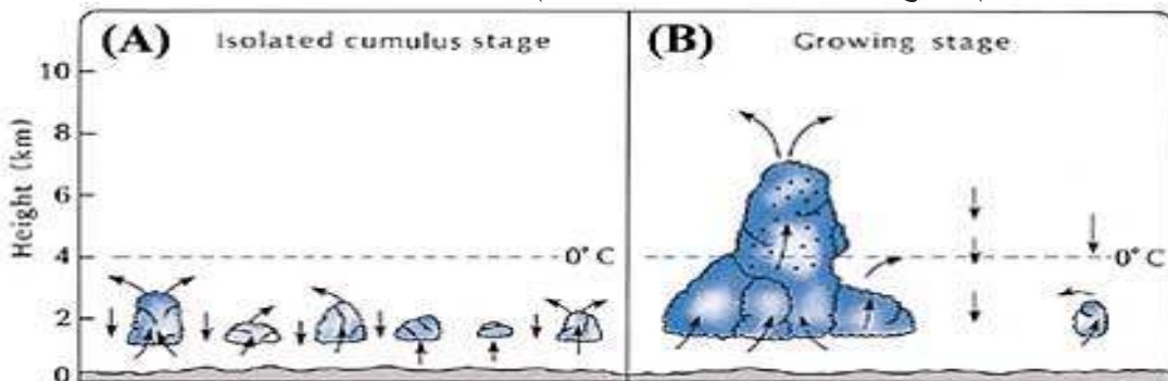
चित्र १९ : (A) Cumulus बादलका स-साना टुक्राहरू
