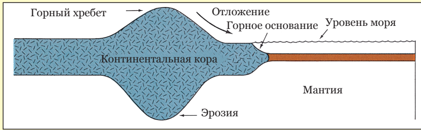
Рис. 9: Еще один рисунок, иллюстрирующий сходство горы с опорой из-за наличия у нее подземной части. ( Earth Science , [”Наука о Земле”], Тарбук (Tarbuck) и Лутгенс (Lutgens), стр. 158.)
