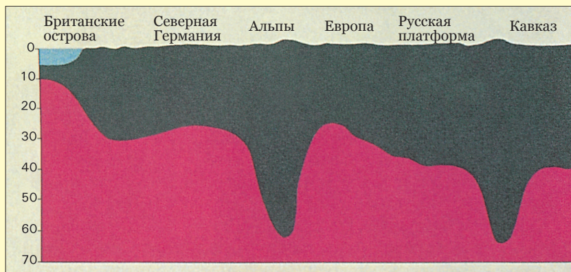
Рис. 8: Схематическое изображение гор в разрезе. Горы, подобно сваям или кольям, уходят глубоко в землю. ( Anatomy of the Earth [”Анатомия Земли “], Кайо (Cailleux), стр . 220.)
