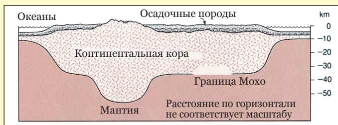
Рис. 7: Горы имеют глубокие “корни”, скрытые под земной поверхностью ( Earth [”Земля”], Пресс (Press) и Сивер (Siever), стр. 413.)
