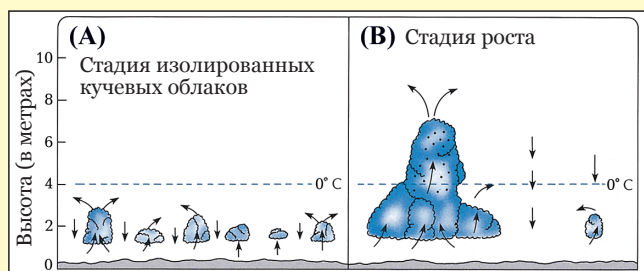
Рис. 19: (А) Небольшие разрозненные фрагменты облаков (кучевые облака). (В) Когда небольшие облака объединяются, восходящие потоки воздуха внутри этого большего облака становятся более сильными, в результате чего облако начинает расти в высоту. Капли воды показаны в виде значков (·). ( The Atmosphere [“Атмосфера”], Энтс (Anthes) и др., стр. 269.)
