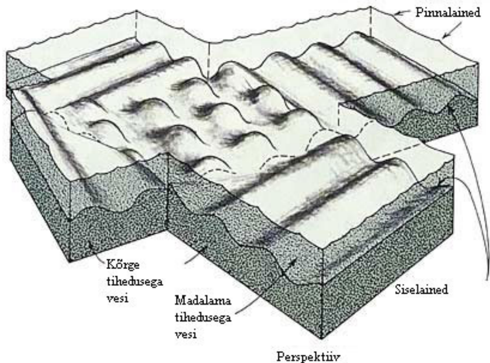
Joonis 16: Siselained kahe erineva tihedusega veekihi vahel. Alumine veekiht on kõrgema tihedusastmega kui ülemine. (Gross. Oceanography. Lk. 208)
