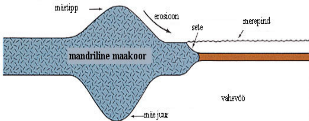
Joonis 2: Veel üks illustratsioon selle kohta, kuidas mäed on maa sees kinni nagu vaiad. (Tarbuck & Lutgens. Earth science. Lk. 104)
