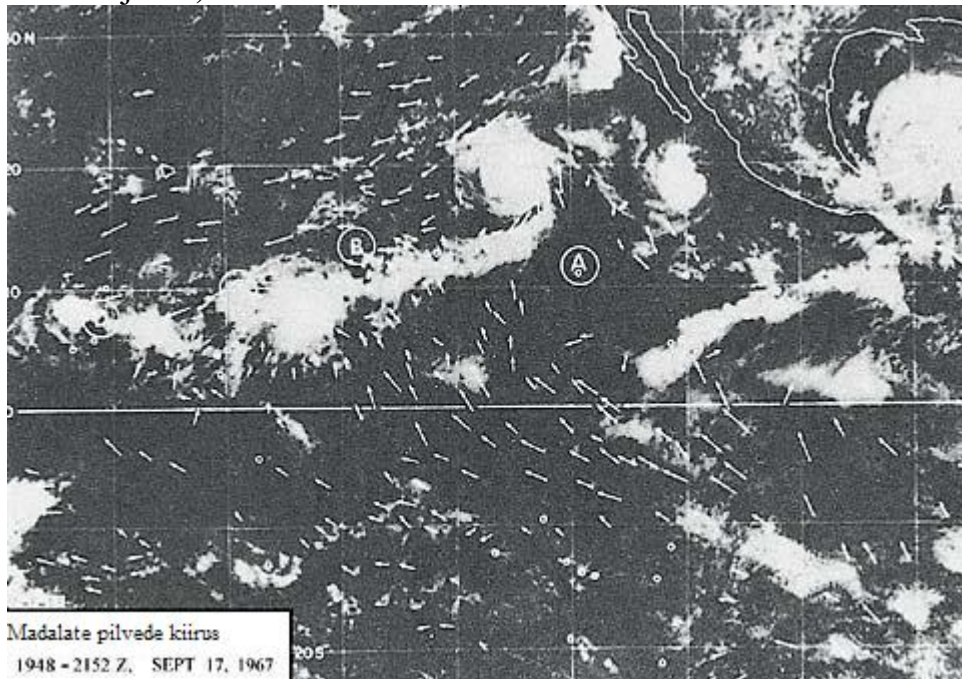
Joonis 17: Pilvede liikumine liitumispirkondadesse B, C ja D; satelliidifoto. Nooled näitavad tuule suunda. (Anderson. The use of satellite pictures in weather analysis and forecasting. Lk. 111)
