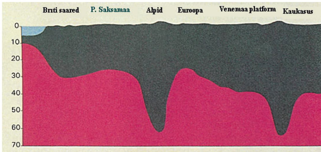
Joonis 1: Skeem mägede ehitusest. (Cailleux. Anatomy of the earth. Lk. 220.)
